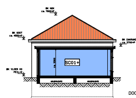
DOORSNEDE
