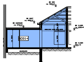
DOORSNEDE
