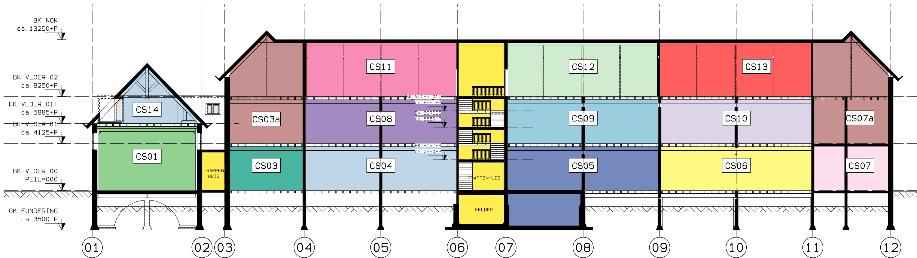
DOORSNEDE A1
