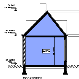
DOORSNEDE
