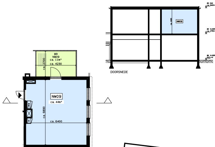
KAPVERDIEPING
