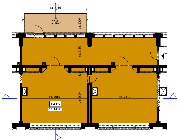
1E VERDIEPING
