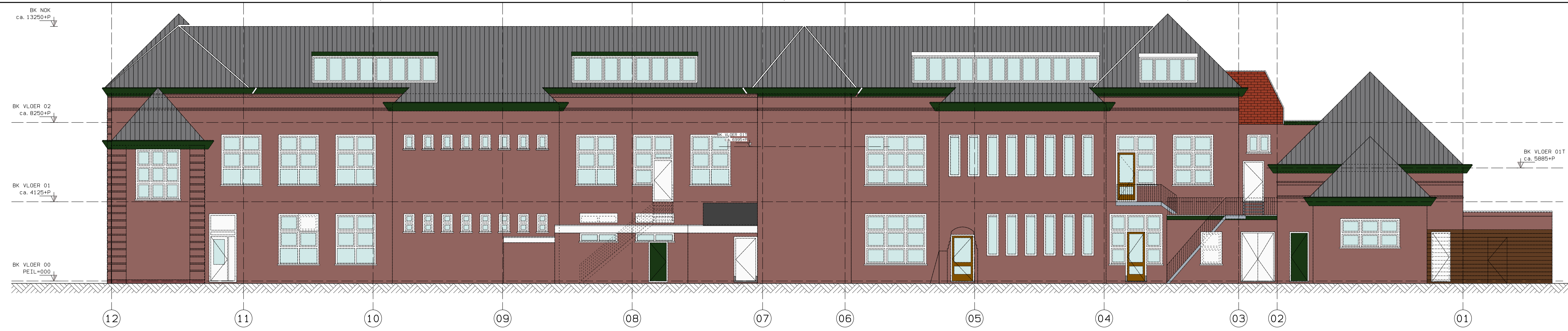
NOORDGEVEL (PLEIN)
