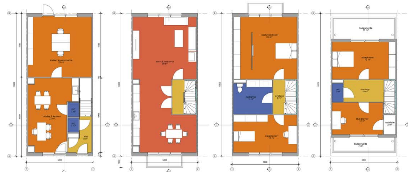
begane grond optie kantoorruimte 72,5m 2
