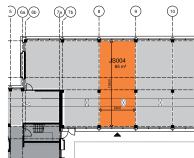
Plattegrond JS004
