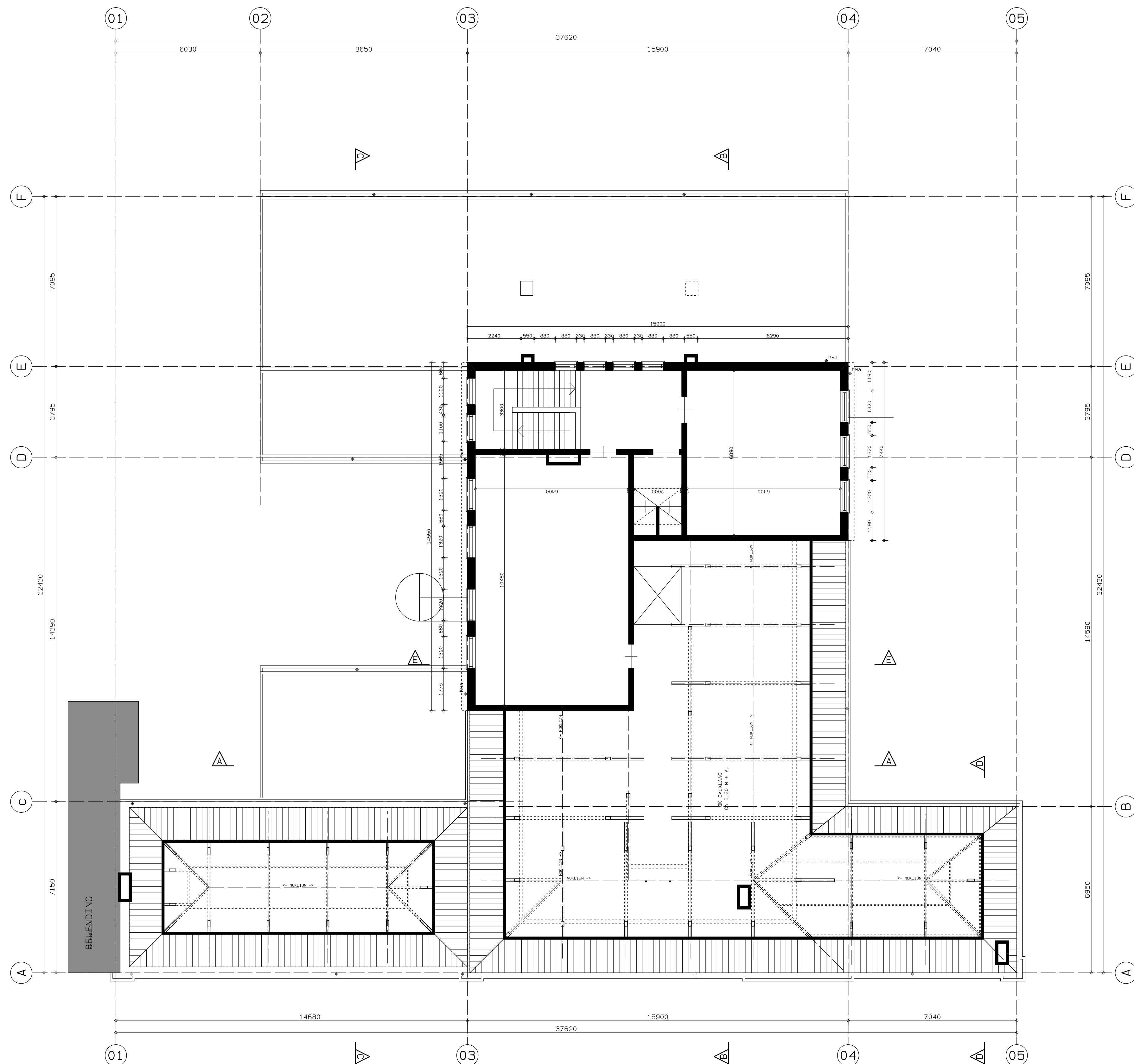
KAP-VERDIEPING BESTAAND
