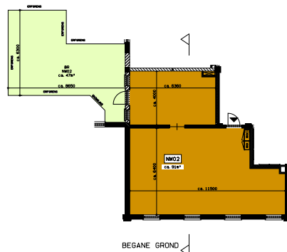
BEGANE GROND
