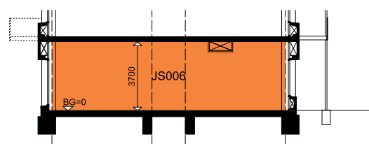
Doorsnede JS006
