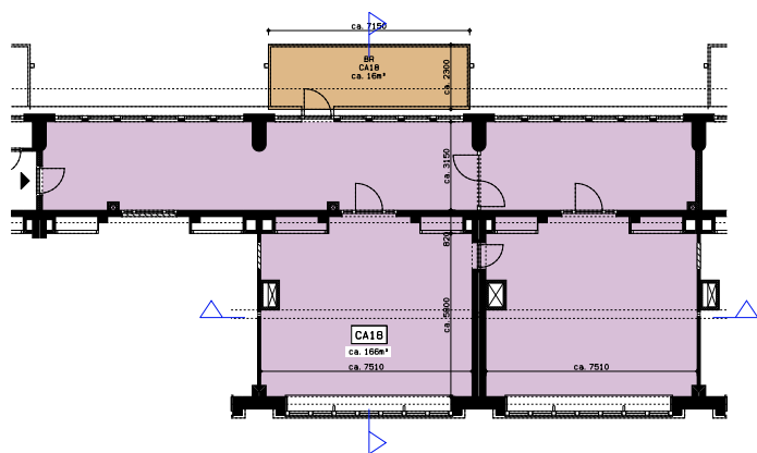
2E VERDIEPING
