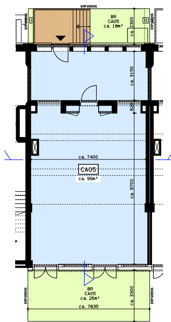
BEGANE GROND
