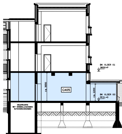
DOORSNEDE
